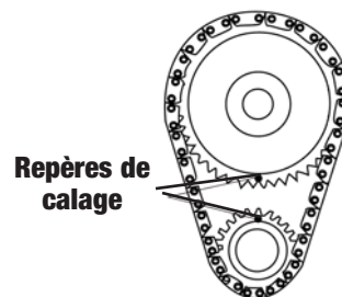
Figure 1 - Alignement des pignons de la chaîne de distribution
